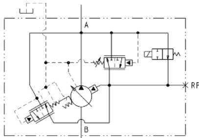
P-C--/H (N.O.) CONTROL
