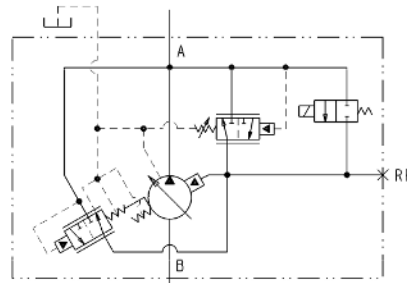
P-K--/H (N.C.) CONTROL
