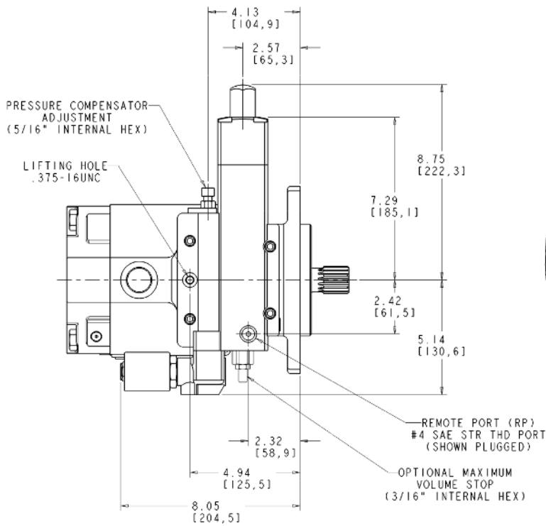
P-C--/H (N.O.) CONTROL
